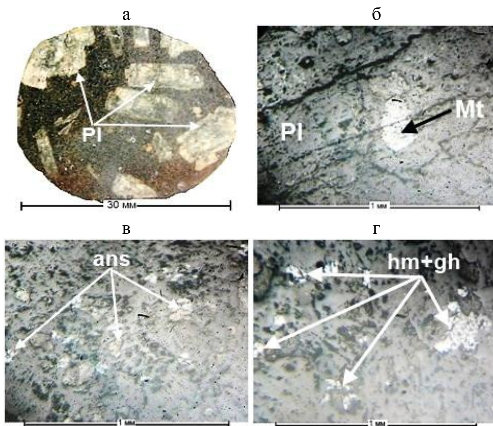
Рис.1.8. Микрофотографии дайки мегаплагиофирового базальта басс. р. Акчасай (АК 8): а – внешний вид (текстура), б – включение магнетита (светлое зерно) в порфирировом выделении плагиоклаза, в – зерна лейкоксена (анатаза) в основной массе порфирита, г – распределение гематита в тонком сочетании с гётитом (светлые зёрна) в основной массе порфирита.
