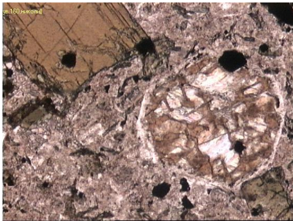
Рис.1.2. Камптонит (АКЗ). а – с крупными фенокристаллами роговой обманки, мелкими порфировыми выделениями псевдолейцита ( d=0,5 мм) окаймленного альбитом. Микрозернистая основная масса сложена призматическими кристаллами роговой обманки, плагиоклаза, листочками биотита, стеклом (?) и изометричными идиоморфными зернами рудного минерала; б – с ксенолитом роговообманкового пироксенита (3x6 см, Каримова, 2018).
