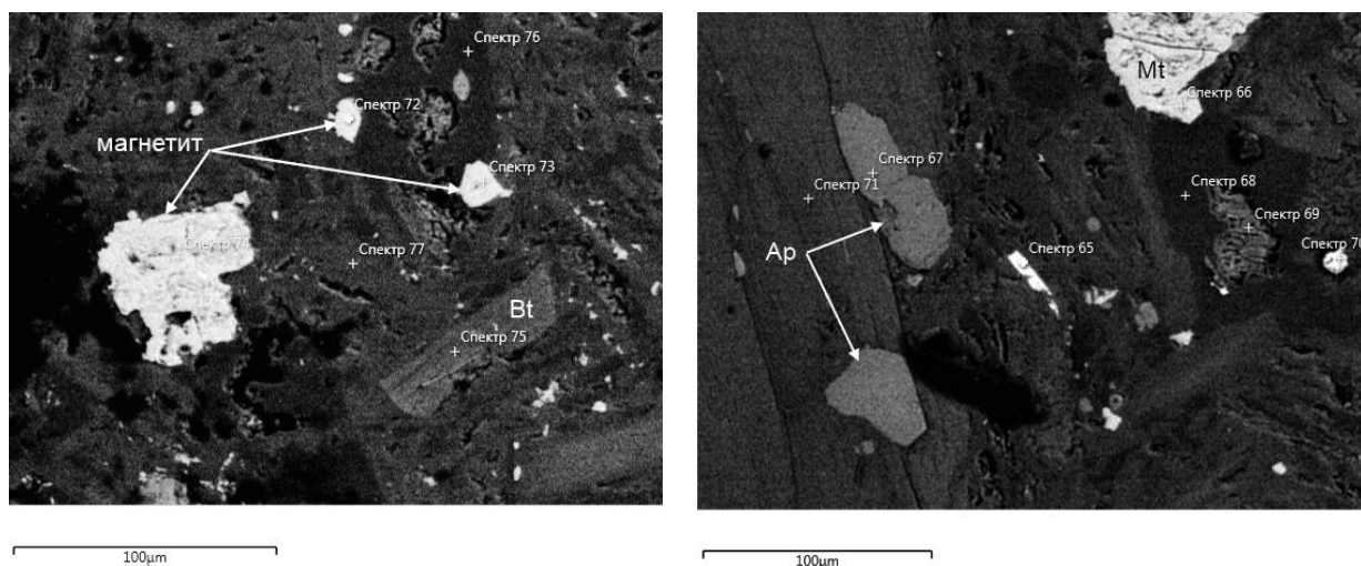
Рис.1.7. Растровые снимки микроминералов в основной массе керсантитовой дайки в басс. р. Акчасай(X-175): а) ксеноморфных зерен селенидов серебра – фрейбергита, который образует реликты ксеноморфных зерен в основной массе, в совместных срастаниях с другими сульфосолями серебра, развитых вокруг зерен сульфидов ранних генераций. Важнейшей особенностью его химического состава является довольно высокая насыщенность серебром 28,98 мас. %. Состав фрейбергитов отличается от теоретического небольшим, но постоянным дефицитом Sb, As; б) выделение корродированного (ксеногенного) зерна гематита, в) загрязненная неправильная форма магнетита и пластинки биотита, г) обилие зерен апатита, магнетита и гематита+тетита. (Сканирующий электронный микроскоп Carl Zeise, с приставкой системы микроанализа Oxford instrument (SEM-EDX). Лаборатория "Физико-химических методов исследования" Центр передовых технологий при Министерстве инновационного развития РУз).
