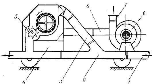
2-расм. Горизонтал қувурда айрилиш зонасига эга бўлган харакатланувчи қурилма
