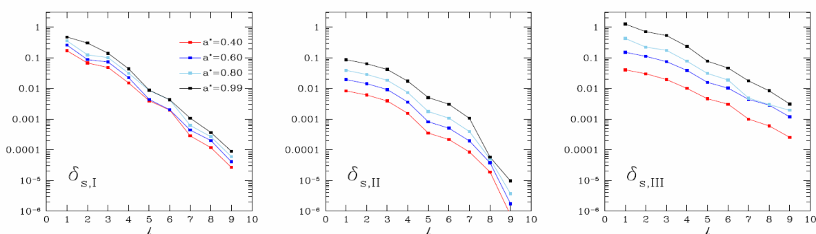
1-расм. Айланувчи қора ўра айланиш параметрларининг турли қийматлари учун сиқилиш параметрининг қатор коэффицентлари даражасига боғлиқлиги.
