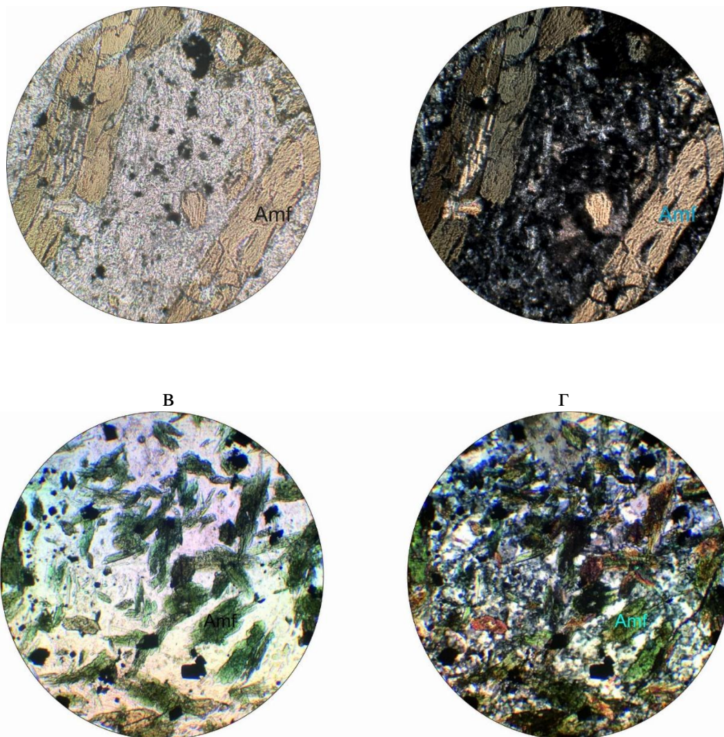
Рис.1.5. Спессартиты (X-169), пр. борт ср. теч. р.Каракиясай. а, в - без анализатора, б, г- с анализатором, увеличение 76 x .
