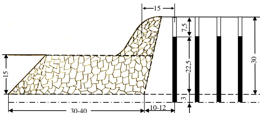
Рис. 1.2. Схема взрывания высоких уступов в зажатой сред
