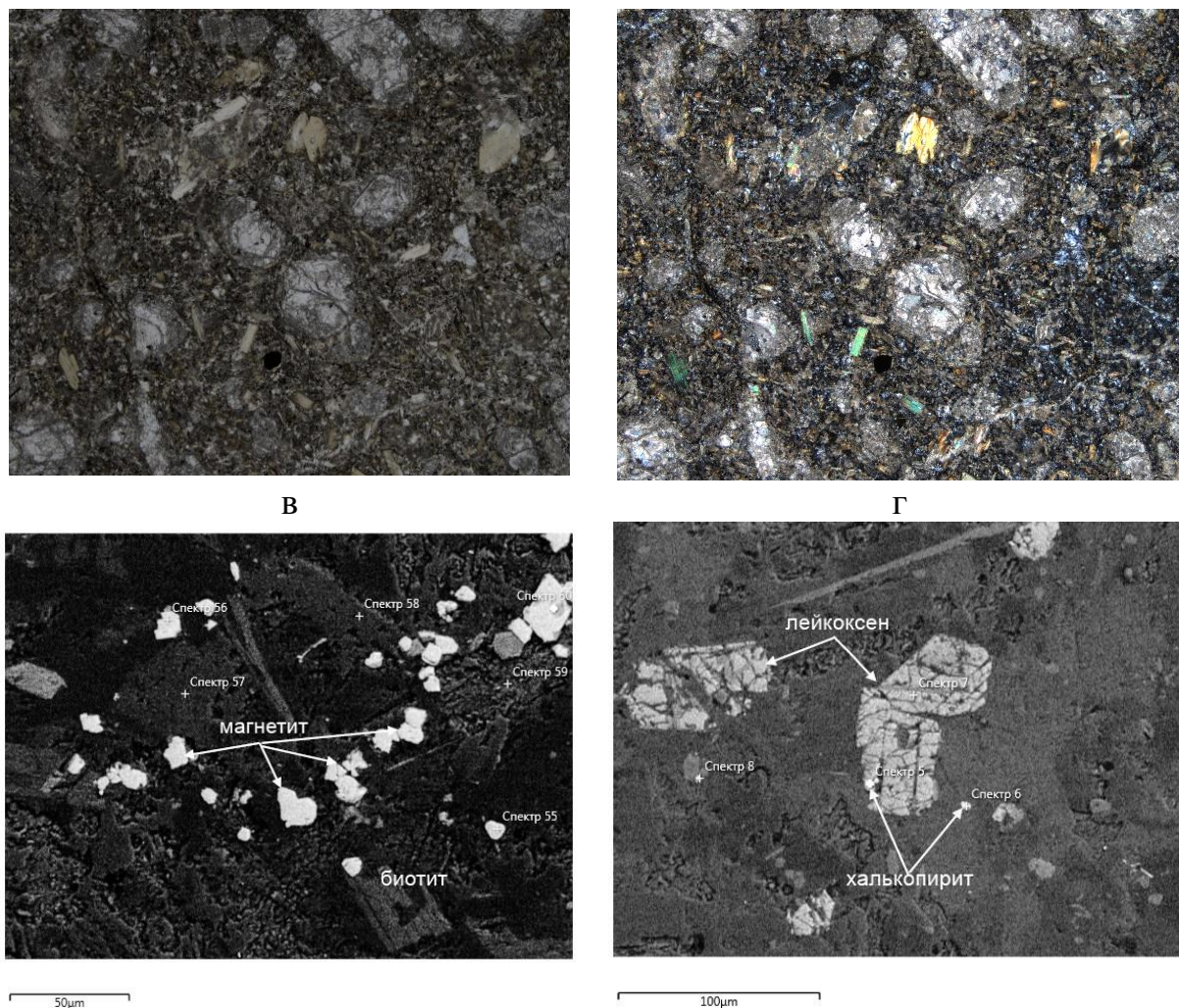
Рис.1.3. Микрофотографии шлифов и растровые снимки микроминералов в основной массе камтомончикитовой дайки в басс. р. Акчасай (АК-3): а) порфировая структура, вкрапленники оливина (при одном николе), б) то же (при двух николях), в) сахаровидный магнетит в основной массе. г) выделения лейкоксена и халькопирита. (Сканирующий электронный микроскоп Carl Zeise, с приставкой системы микроанализа Oxford instrument (SEM-EDX). Лаборатория "Физико-химических методов исследования" Центр передовых технологий при Министерстве инновационного развития РУз).
