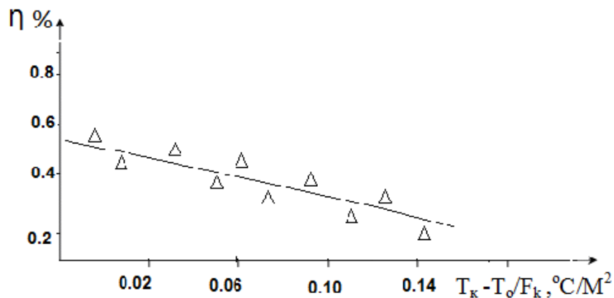
Рис. 2. Тепловой КПД энергетического модуля солнечного параболоцилиндрического коллектора, зеркальной площадью 8, 75 м 2 .
