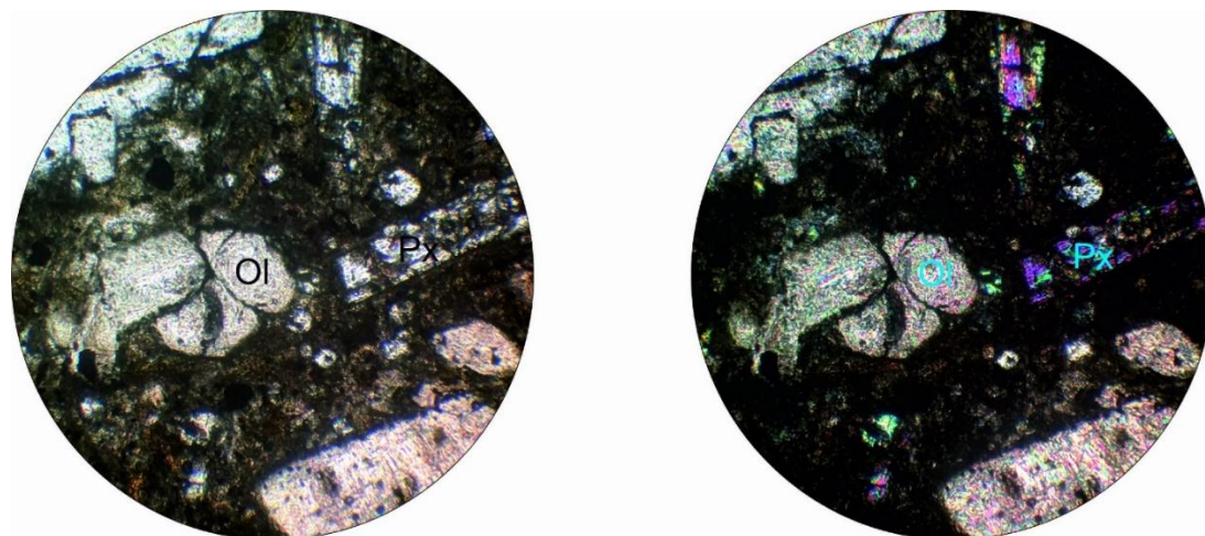
Рис.1.1. Микрофотографии шлифов мончикитов (АК 6). Структура порфировая с скрытокристаллической, гиалопилитовой основной массой. Минеральный состав: порфировые выделения составляют до 40% от всей породы. Представлены оливином, моноклинной пироксеном, биотитом. Увел. 76 раз.
