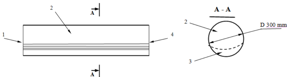
1- расм. Таклиф этилаётган янги қувур схемаси.
