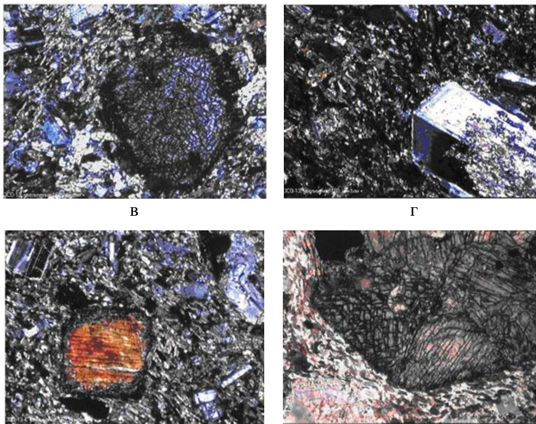
Рис.1.4. Одинит. Структура породы порфировая (Каримова Ф.Б.,2018).
