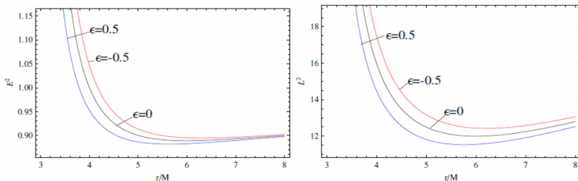
2-расм. Деформация параметрининг турли қийматлари учун қора ўралар атрофида доиравий орбита бўйлаб ҳаракатланаётган зарраларнинг энергияси (чапда) ва импульс моментларининг (ўнгда) радиал ўзгариши.
