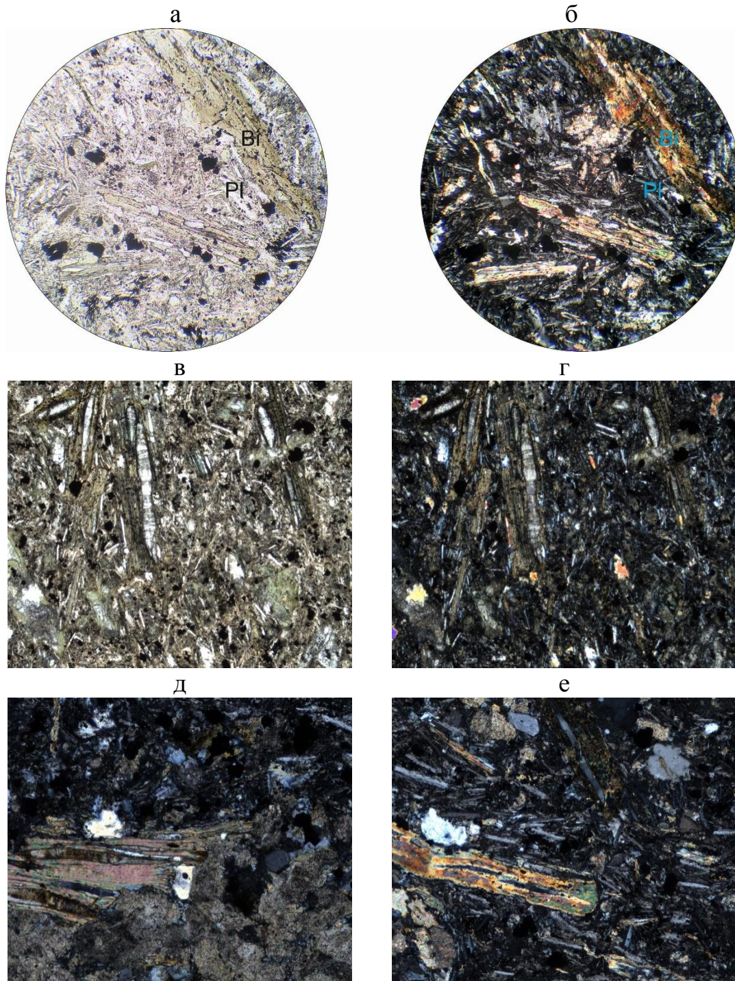
Рис.1.6. Керсантит (X-175), лев. борт р. Акчасай. а) без анализатора б) с анализатором, увеличение 76 x .
