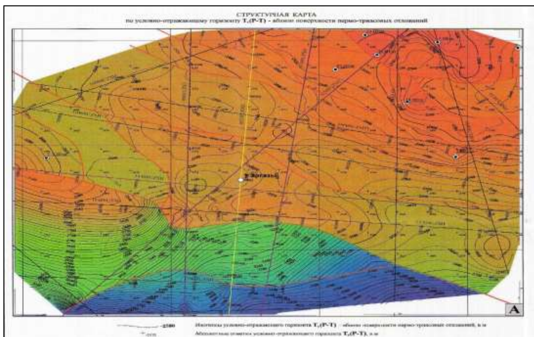
Рис. 3. Структурная карта по условно-отражающему горизонту T_v(P-T) вблизи поверхности пермо-триасовых отложений
