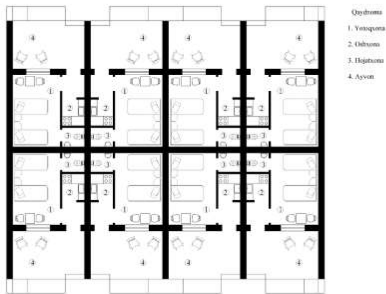
6-Rasm Yusuf Hamadoniyy ziyoratgohiga ziyorat va davolanish uchun kelgan ichki va tashqi turistlar uchun yangi ekoturistik mehmonxonlarning tarh rejasi taklif loyihasi
