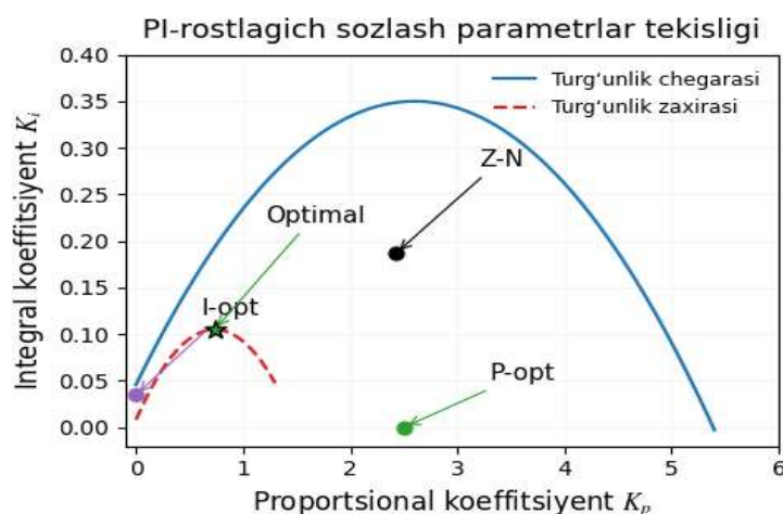
6-rasm. P, I va PI rostlagichlarining bosqichli munosabat taqqoslama grafigi. PI rostlagich ( K_p = 0.734 , K_i = 0.105 ) statik xatolikni nolga tushirib, 1.8 s ichida \leq 3.1\% ortiq o'tish bilan barqarorlikka erishadi.
