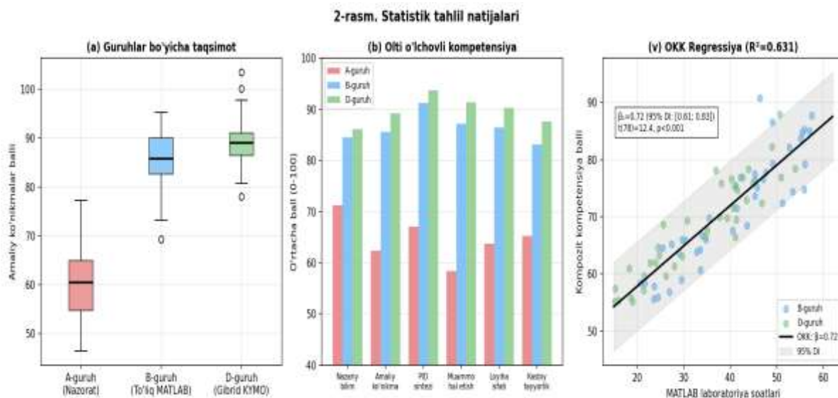
2-rasm. Statistik tahlil: (a) guruhlar bo'yicha amaliy ko'nikmalar balllarining taqsimoti; (b) olti o'lchamli kompetensiya o'rtachalari; (v) 95% bashorat bandi bilan MATLAB lab soatlari va kompetensiya balli o'rtasidagi OKK regressiyasi.
