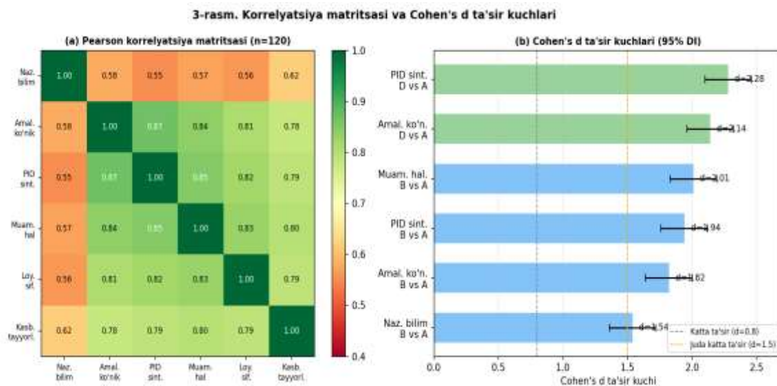
3-rasm. (a) olti kompetensiya o'lchami bo'yicha Pearson korrelyatsiya matritsasi ( n=120 ); (b) guruh taqqoslashlari uchun Cohen's d ta'sir kuchlari — barcha d > 1,5 (istisno darajali).
