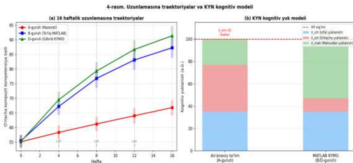
4-rasm. (a) Intervensiya markerlari va 95% DI bant bilan 16 haftalik uzunlamasına kompetensiya traektoriyalari; (b) MATLAB o'rganish mexanizmini tushuntiruvchi KYN-asosida kognitiv model.
