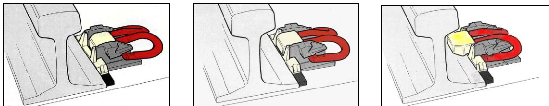
1-rasm. «Pandrol Fastclip» biriktirgich montaji sxemasi
