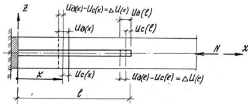
Рис. 1. Расчетные схемы соединений на клеенных стержнях с упором арматурного стержня в торец
