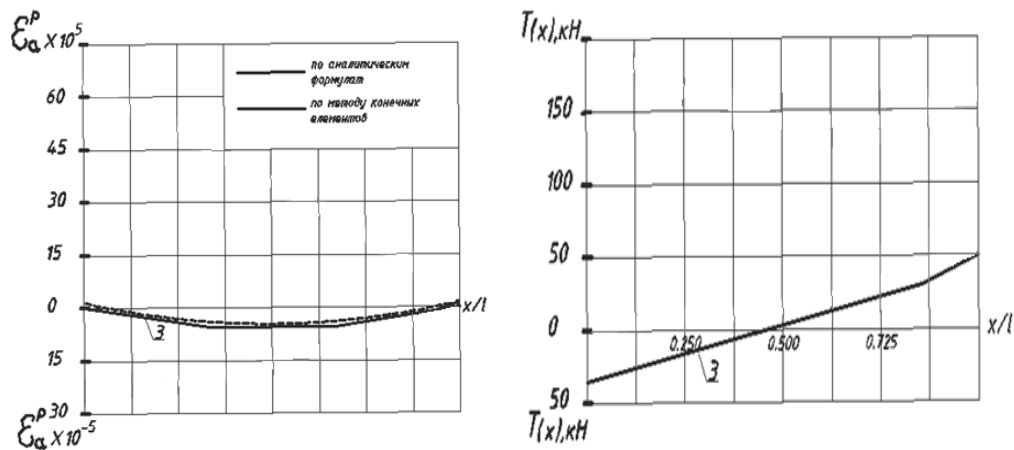
Рис. 2. Распределение относительных деформаций (а) и силы сдвига (б) по длине вклеенного стержня при сжатии с упором стержней в торец.
