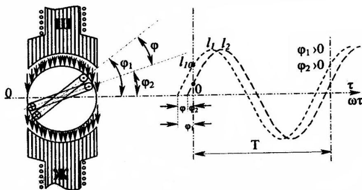
2- rasml. Őzgaruvchan tokning boshlang'ich fazasi va faza siljishi.
