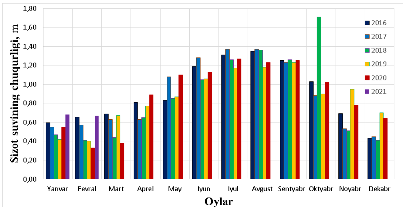
2-rasm. Yil va oylar bo'yicha yer osti sizot suvining ko'tarilish va pasayish diagrammasi
