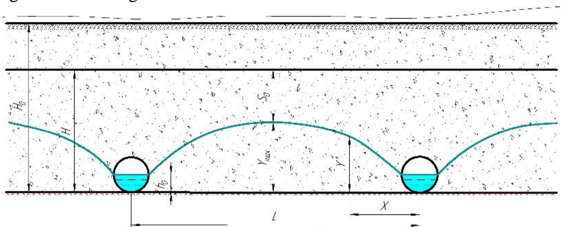
3-rasm. Mukammal drenajning hisob sxemasi
