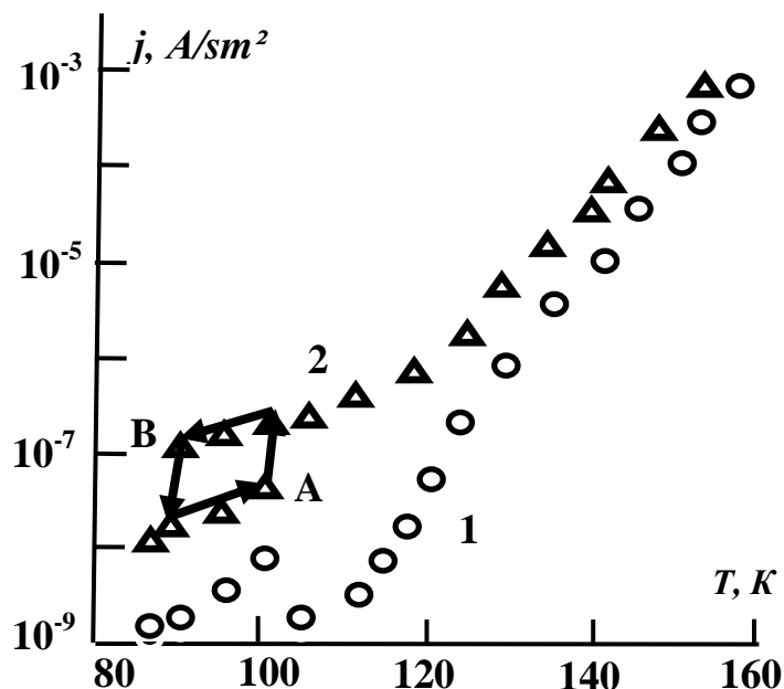
Рис. 3. Температурные зависимости темнового (кривая 1) и фототоков (кривая 2) в ПФИК с фотоприемником из Si<Pt> .
