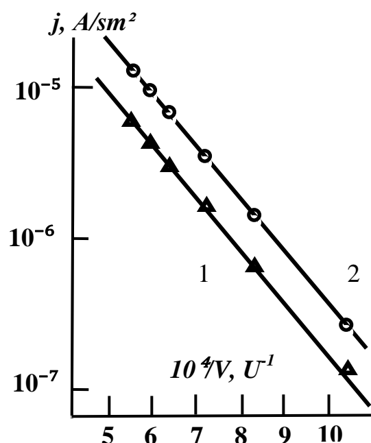
Рис. 1. Вольтамперные характеристики автоэлектронной эмиссии с GaAs: 1 - в темноте, 2 - при освещении.
