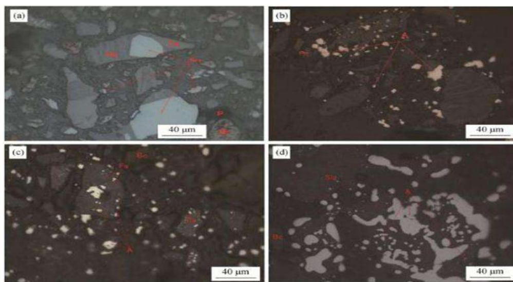
3-расм. Турли ҳароратларда: (a) 600 °C; (b) 800 °C; (c) 900 °C; (d) 1000 °C тикланган донатор зарраларнинг оптик микроскопияси. А - металли фаза; Вс – қора кўмир; Frr - феррит; Fa - фаялит; P - тешиқлар; Slg - шлак; Hd - геденбергит
