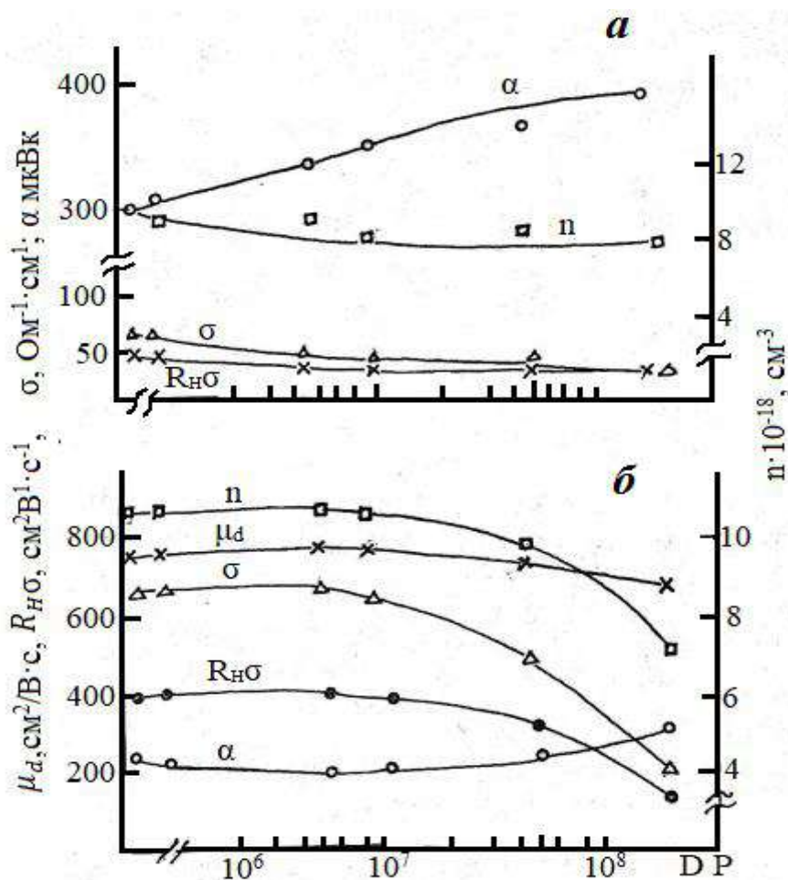
Рис.1. Влияние \gamma – облучения на параметры пленок n - \text{PbTe} сконденсированных при 340 \text{ }^\circ\text{K} (а) и 370 \text{ }^\circ\text{K} (б). ( \circ - \alpha , \Delta - \sigma , \square - n , \bullet - R_H \sigma , \times - \alpha^2 \sigma , \times - \mu_d ).
