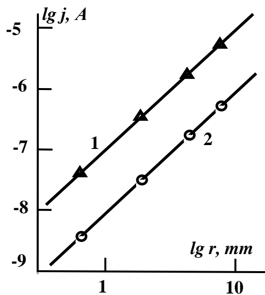
Рис. 2. Зависимость автоэлектронного тока от радиуса отверстия в диэлектрической прослойке. V, кВ: 1 - 1,5; 2 - 1.
