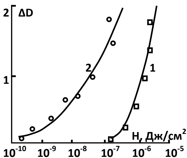
Рис. 4. Характеристическая кривая (абсолютной величины оптической плотности изображения от экспозиции) фотографического процесса в ПФИК для спектрального диапазона длин волн \lambda = 2,6 \div 4,2 мкм: 1 – без усиления инфракрасного изображения; 2 – усиленное инфракрасное изображение с помощью ЭП-16.
