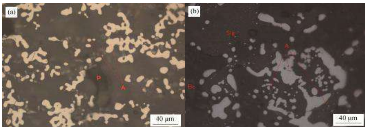
4-расм. Кўмирнинг турли дозаларида: а) 15%; (b) 25% тикланган донатор зарраларнинг оптик микроскопик тасвирлари. А - металли фаза; Slg - шлак; Вс – қора кўмир; P - тешиқлар
