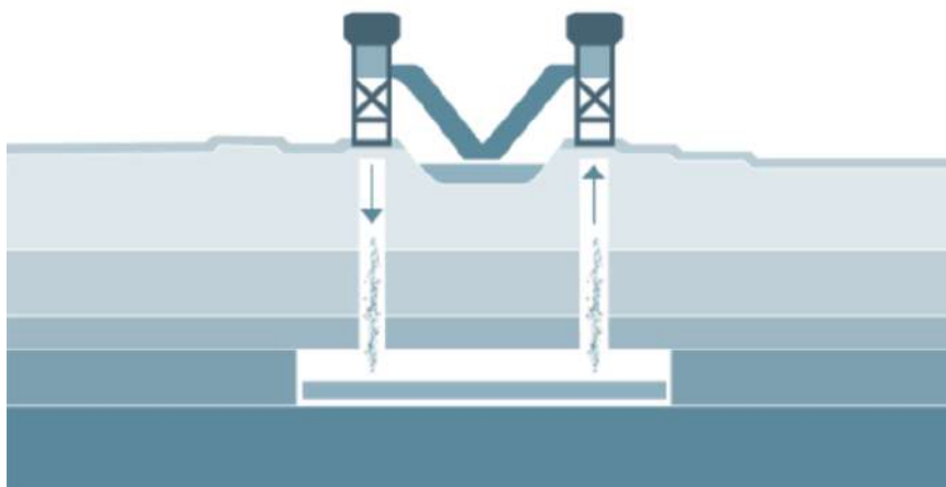
2-rasm. Kaliy rudalarini yer ostida ishqorli eritish usuli.
