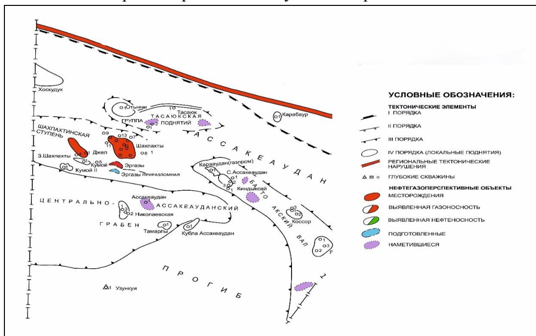
Рис. 2. Схема расположения нефтегазоперспективных структур Южного Уstyурт
