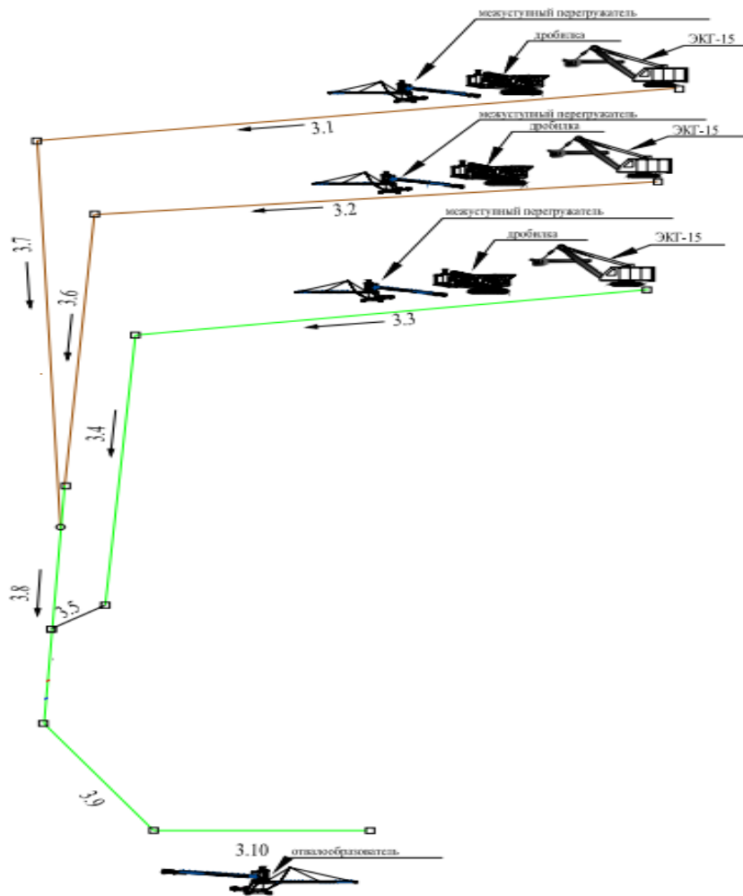
Рис.1. Схема расположения вскрышных конвейеров на линии ЦПТ в разрезе Ангренский [8,9]
