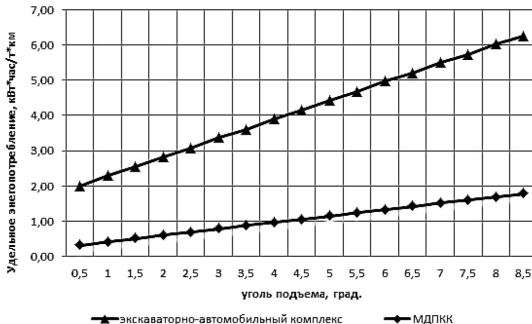
Рис 2. Зависимость удельного энергопотребления от изменения высоты подъёма для экскаваторно-автомобильного комплекса и комплекса МДПКК в условиях разреза Ангренский
