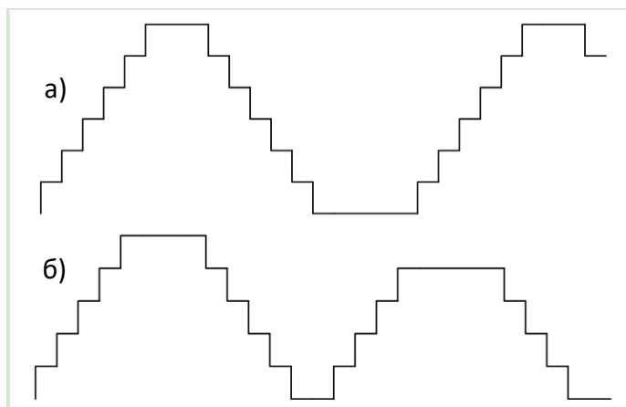
Рис. 2 - Картины МДС при \gamma=8
