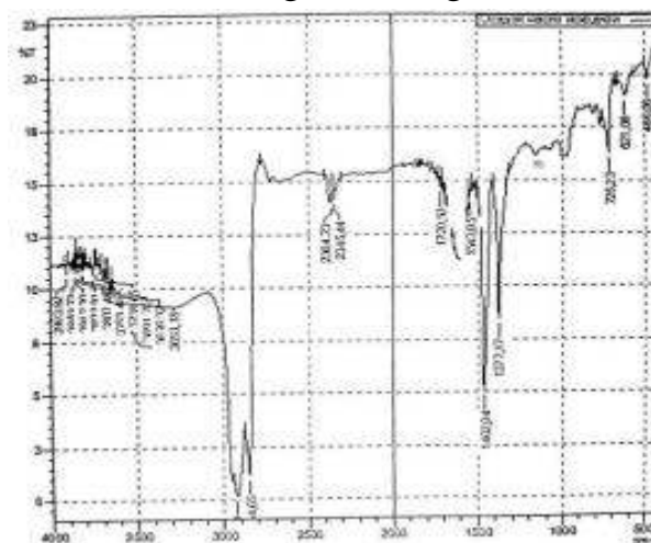
1-rasm. Gidravlik suyuqliklarning infraqizil spektrlari
