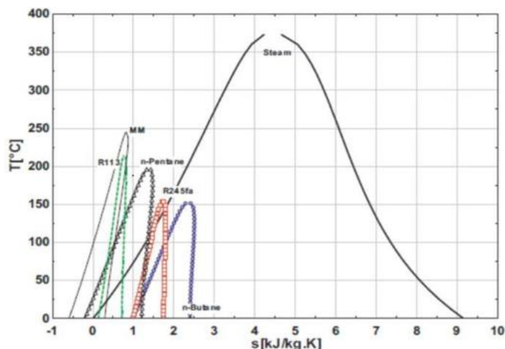
Рис. 2. T-s диаграмма воды и некоторых органических рабочих тел.
