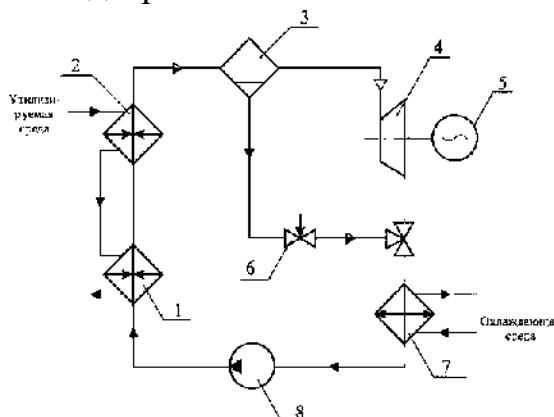
Рис. 3. Схема цикла Калины:
