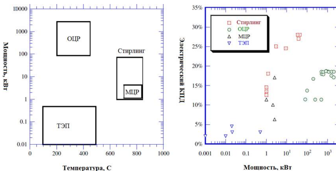
Рис. 4 . Сравнение технологий преобразующих тепловую энергию в электрическую.
