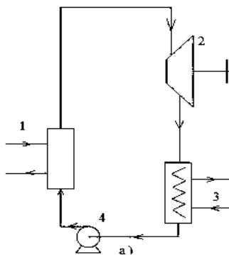
Рис. 1. Схема органического цикла Ренкина:
