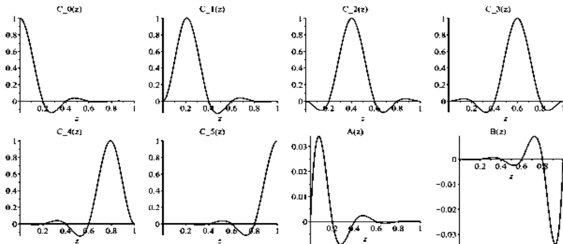
Рис. 1. Графики оптимальных коэффициентов \overset{\circ}{C}_\beta(z) , \beta = \overline{0,5} и \overset{\circ}{A}(z) , \overset{\circ}{B}(z) оптимальной интерполяционной формулы (1.64).
