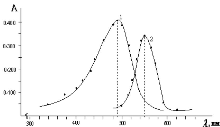
Рис.1. Спектры поглощения реагента HR (1) и его комплекса со свинцом (2)
