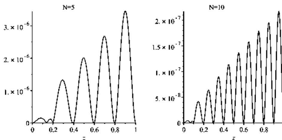
Рис. 2. Графики абсолютных ошибок \left| \varphi_1(z) - \overset{\circ}{P}_{\varphi_1}(z) \right| для случаев N = 5 и N = 10 .
