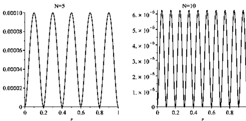
Рис. 3. Графики абсолютных ошибок \left| \varphi_2(z) - \overset{\circ}{P}_{\varphi_2}(z) \right| для случаев N = 5 и N = 10 .
