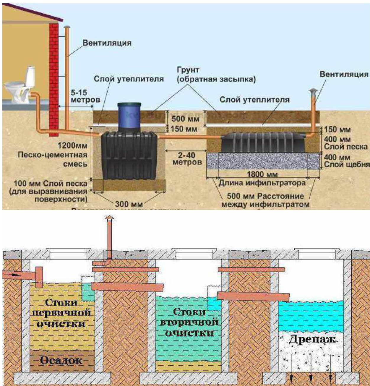
4-рasm. Septik qurilmalarni izolyatsiya qilish sxemasi
