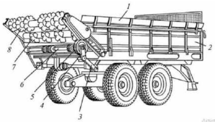
Рис. 1 Разбрасыватель органических удобрений РОУ-б:
