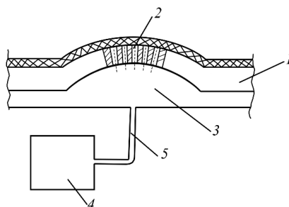
Рис.1. Нижняя подушка устройства вакуумного формообразования деталей одежды:
