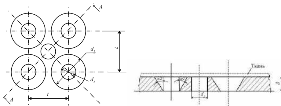
Рис. 3. Элементарная ячейка с перфорациями в пределах толщины 8 нижней подушки устройства для формообразования объемных деталей одежды методом вакуумирования; -узел конусности; t – шаг перфораций, d_1 , d_2 – соответственно диаметры входного и выходного отверстия.
