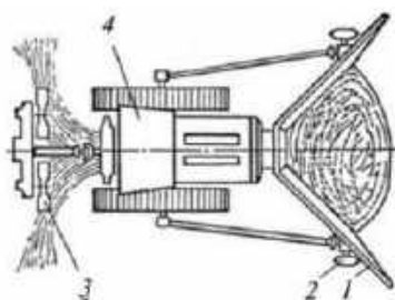
Рис. 2 Разбрасыватель РУН-15Б:
