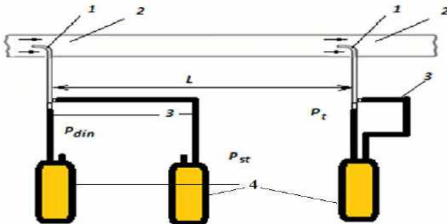
1-rasm. Pito trubkasi va uni quvur va mikromanometrға ulash sxemasi. 1- Pito trubkasi; 2-quvur; 3-rezina shlang; 4-mikromanometr
