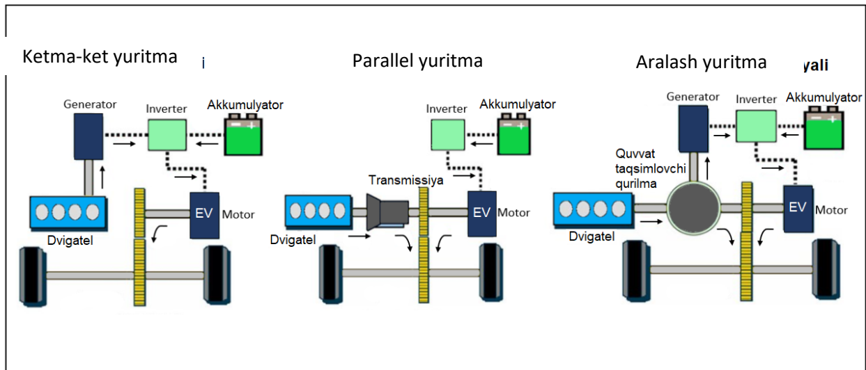
3-rasm. Gibridd elektr transport vositalarining konfiguratsiyalari 42
