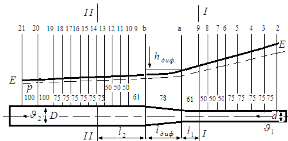
Рис.1. Схема для определения потерь напора в диффузоре
