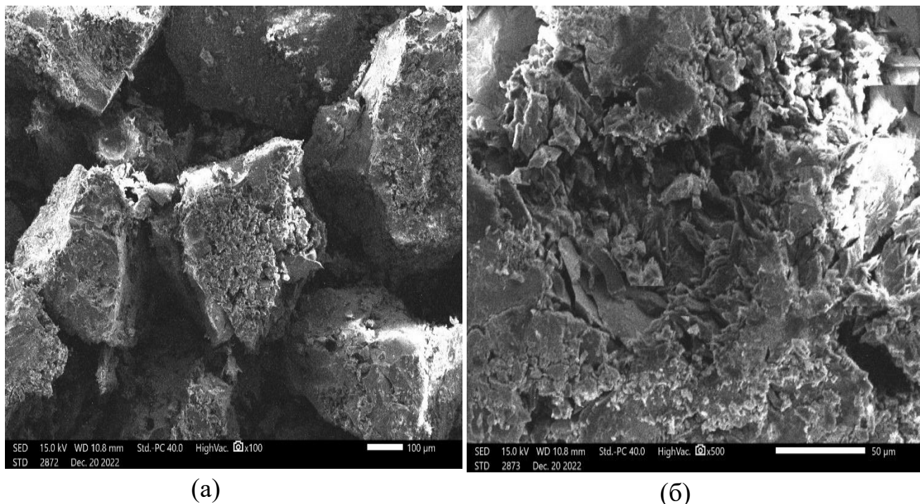
Рисунок 4. СЭМ-изображения бетона, модифицированного серо-2,4-динитрофенилгидразином, при различных увеличениях: (а) 100 мкм и (б) 50 мкм.
