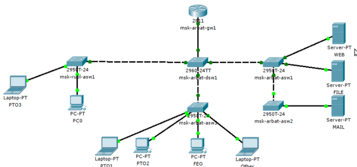
Рис. 1. Конфигурация лабораторной работы 5: статическая конфигурация маршрутизатора 3 (в режиме моделирования)
