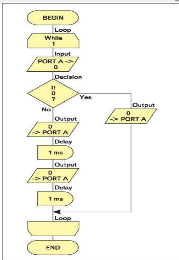
Рис. 2. Блок-схема, созданная во Flowcode
