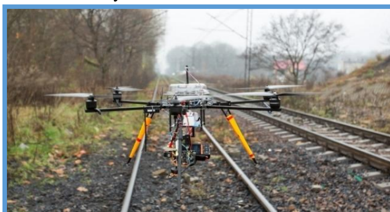
3-расм. Учувчисиз учиш дефектоскоп аппарати
