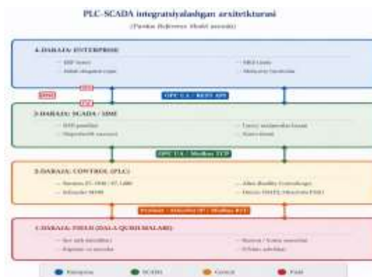
1-rasm. PLC-SCADA integratsiyalashgan arxitekturasini (Purdue modeli)
